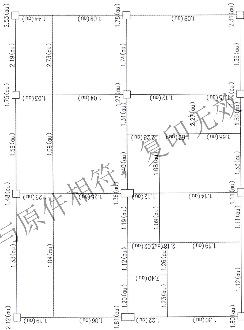
附图 3-1 一层梁、柱安全性验算结果
