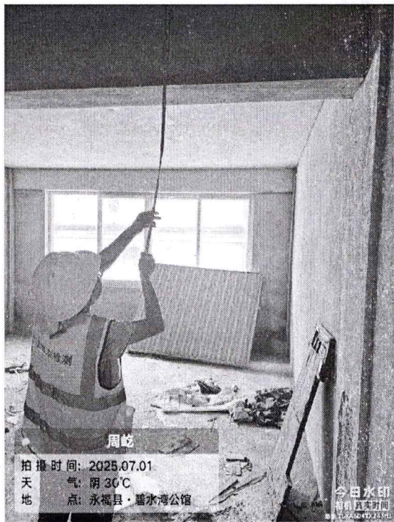
附照片 2-1 梁构件尺寸检测现场照片
